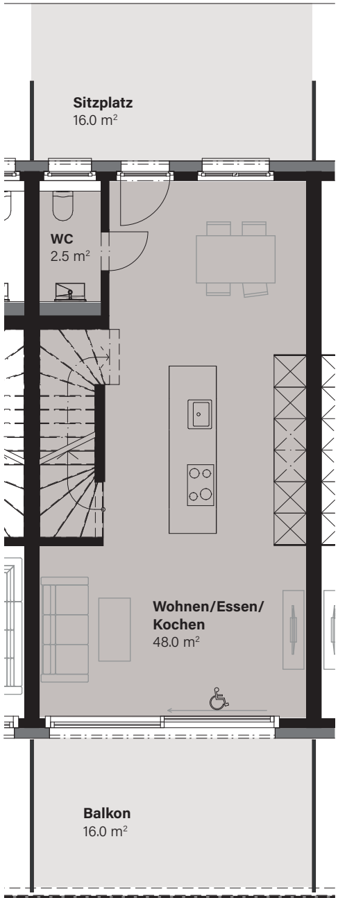
OBERGESCHOSS
