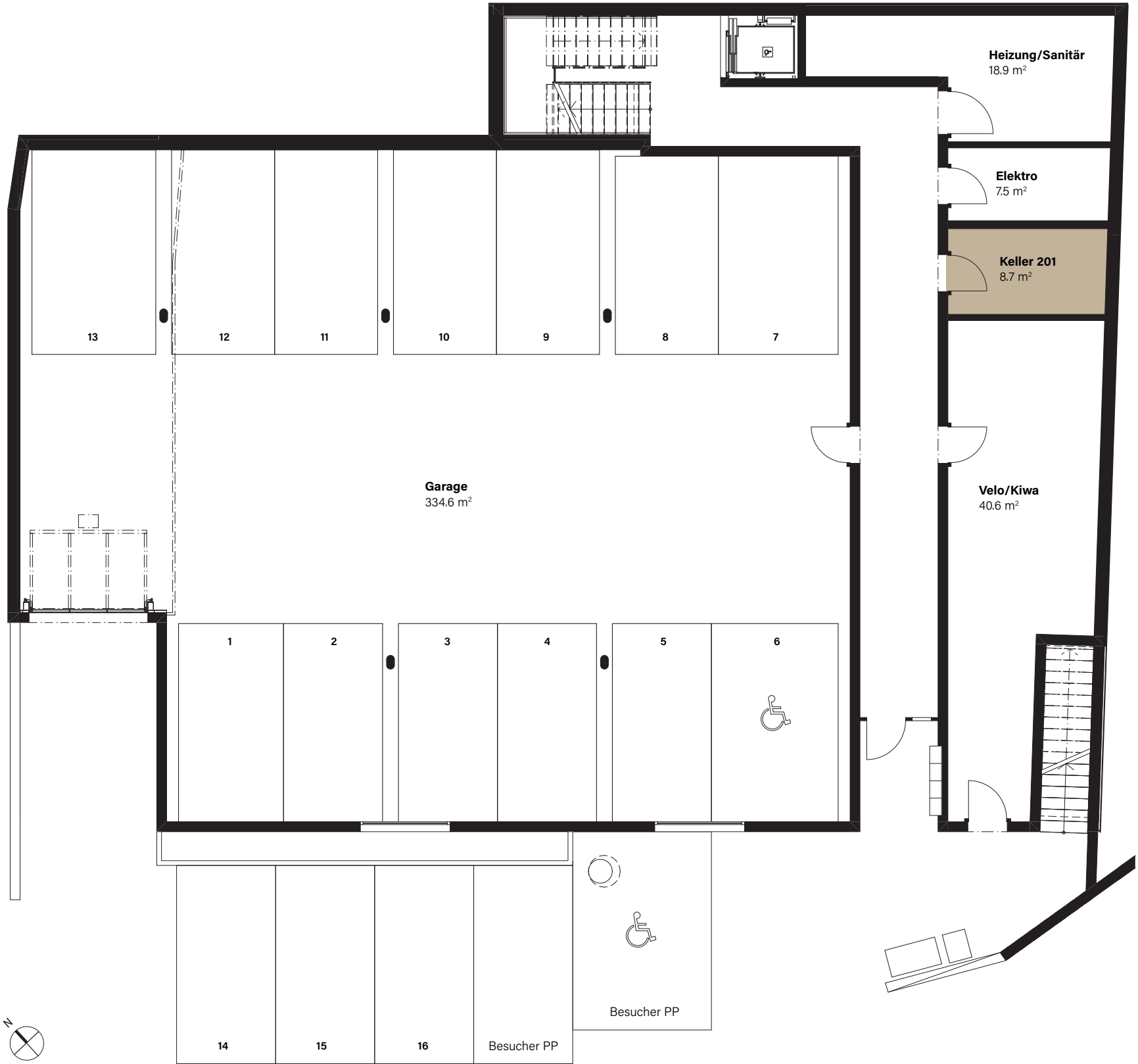
UNTERGESCHOSS
